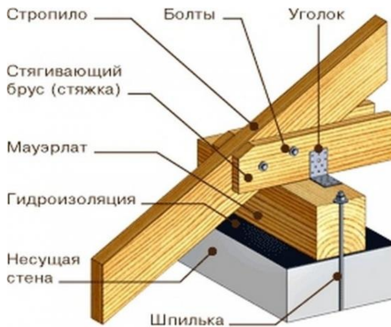
Рис. 1 Крепление мауэрлата к несущей стене
