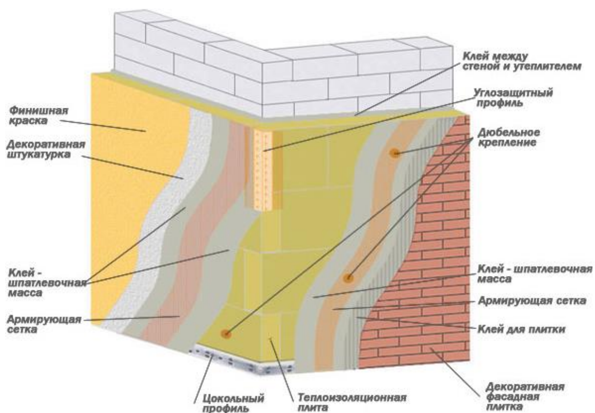
Рис. 2. Состав слоёв отделки фасадов зданий
